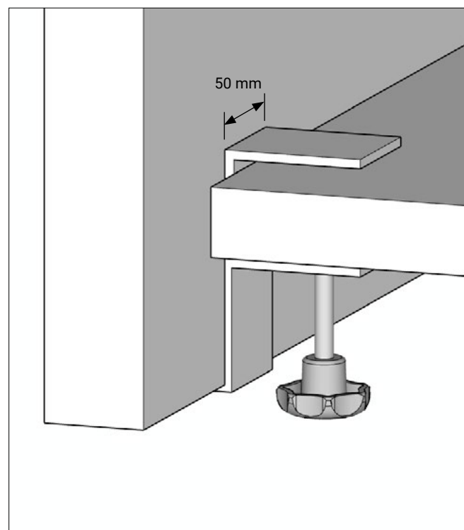
FLZTV Tischhalter-Set vorgesetzt
