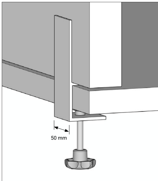
FLZTA Tischhalter-Set aufgesetzt
